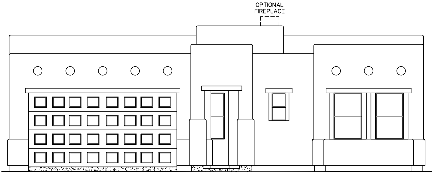
ELEVATION A
